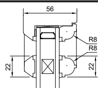
Profil standard SASH OVOLO R8
