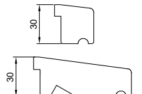
Profil standard SASH LAMB
