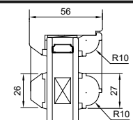
Profil standard SASH OVOLO R10
