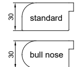
Profil standard SASH OVOLO R10
