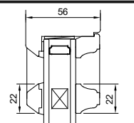
Profil standard SASH LAMB
